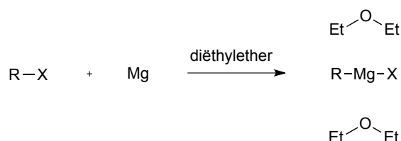
Figuur 5.43 Synthese van het Grignardreagens
