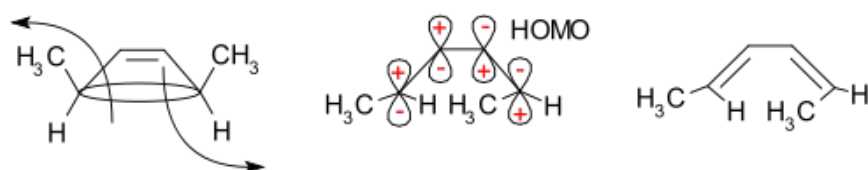
Figuur 5.49 Van rechts naar links: beide eindgroepen conroteren tijdens de vorming van eindproduct
