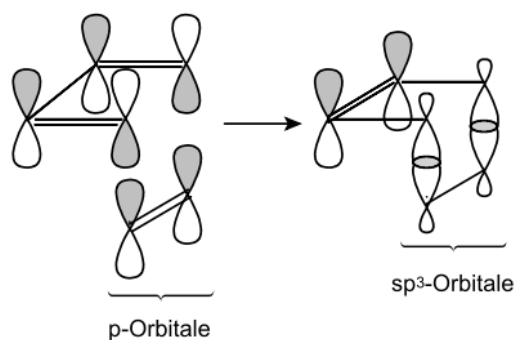
Figuur 5.52 HOMO van dieen reageert met LUMO van diënofiel.
