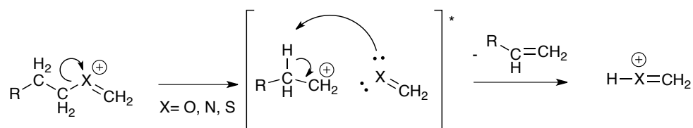
Figuur 7.13 Ontledingen van oxonium, iminium, etc. ionen (ontstaan uit ethers, aminen, etc.)
