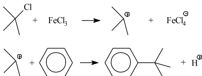
Figuur 5.36 Alkylering: Het is ook mogelijk om secundaire en tertiaire halogeenalkanen te activeren.
