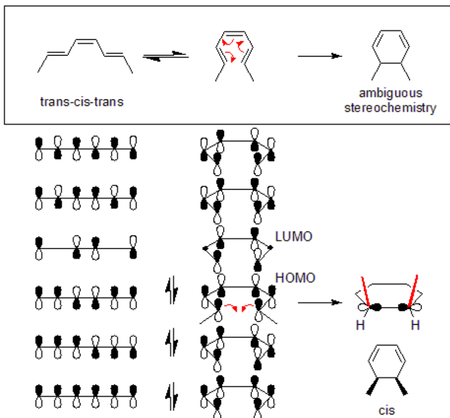
Figuur 5.50 Deze figuur laat zien hoe bij een open-keten-systeem met 6 \pi -elektronen het eindproduct ontstaat. In het bovenste deel van de figuur wordt geen rekening gehouden met de symmetrie van de betrokken orbitalen, in het onderste deel wel.
