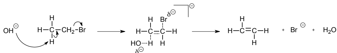
Figuur 5.29 Een voorbeeld van E2-eliminatie: dehalogenering. Vergelijk ook met het S N 2-mechanisme.
