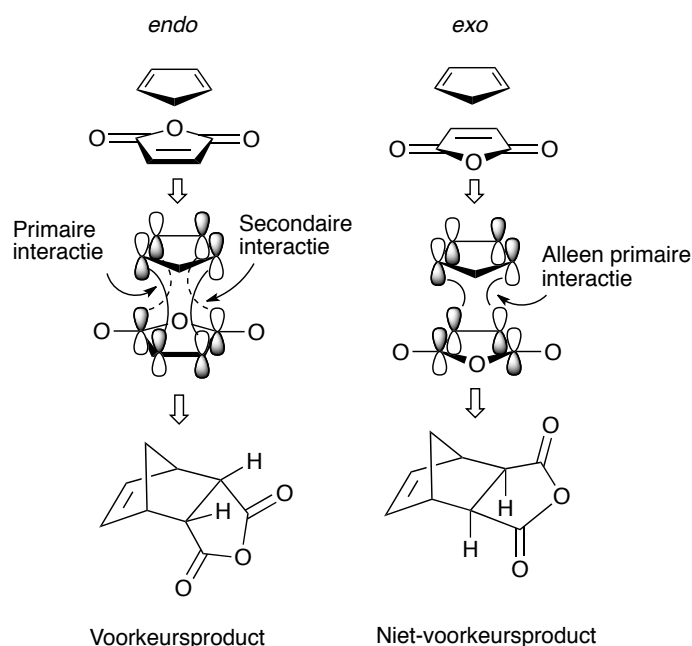
Figuur 5.56 Reactie tussen cyclopentadien en maleïnezuuranhydride. Links is de endo -oriëntatie te zien, die extra stabiliserende overlap toelaat, terwijl bij de exo -oriëntatie rechts geen secundaire interactie mogelijk is.
