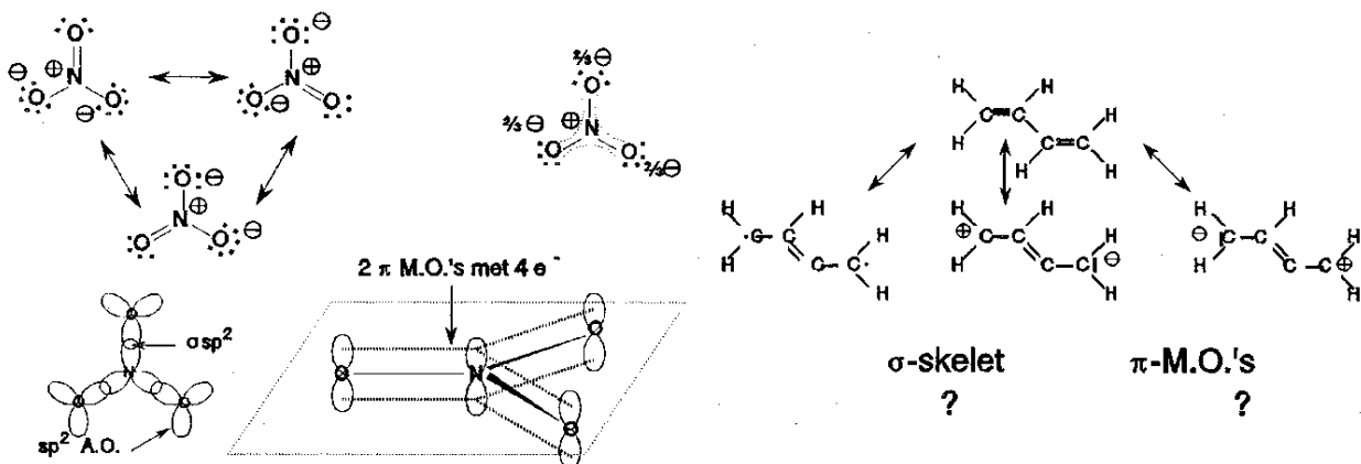
Figuur 3.19 Mesomerie in nitraat en butadiëen
