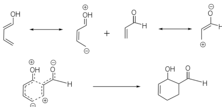
Figuur 5.53 Het dieen (links) en diënofiel (rechts) vormen slechts één structuurisomeer (de ortho -variant) en niet de andere mogelijkheid (de meta -variant).
