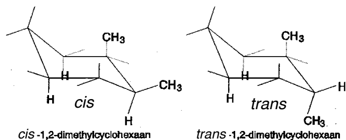
Figuur 5.12 Ringstructuren: cis en trans
