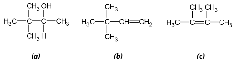
Figuur 5.45 Dehydratie van 3,3-dimethylbuta-2-ol
