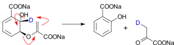
Figuur 5.48 De omzetting van isochorismaat in salicylaat en pyruvaat is een (gekatalyseerde) pericyclische reactie
