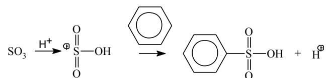
Figuur 5.35 Sulfonering: SO 3 activeren met H 2 SO 4 .
