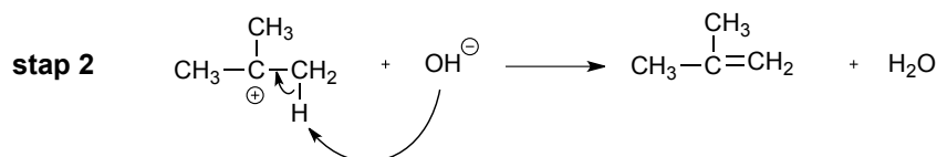
Figuur 5.28 Het mechanisme van E1-eliminatie. Vergelijk ook met het S N 1-mechanisme
