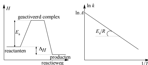
Figuur 4.20 Bepaling activeringsenergie
