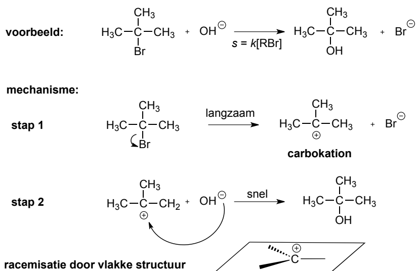
Figuur 5.18 Samenvatting van S N 1-reacties
