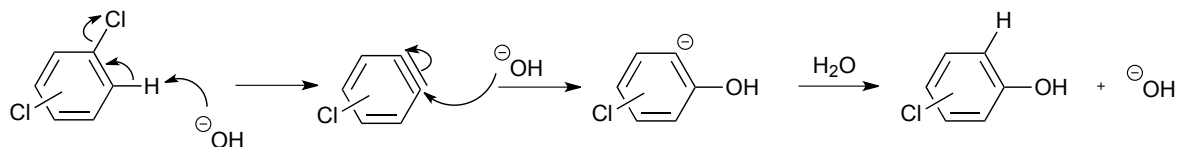
Figuur 5.23 Een alternatief mechanisme met benzyn als intermediair
