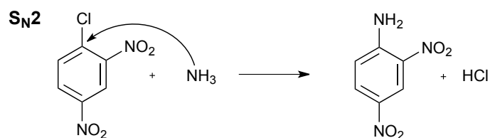
Figuur 5.21 Samenvatting van aromatische substituties
