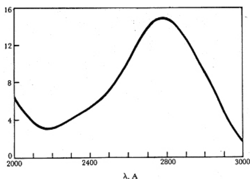
Figuur 7.4 Het UV-spectrum van acetone
