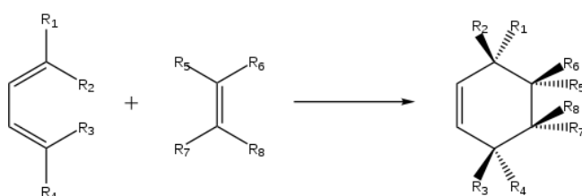
Figuur 5.54 Behoud van configuraties
