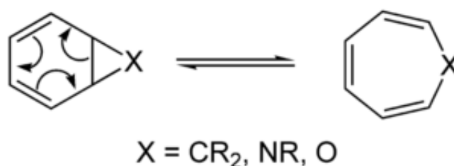
Figuur 5.47 Voorbeeld van een pericyclische reactie
