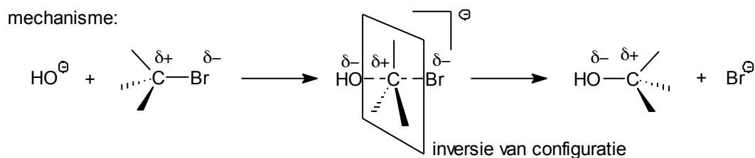
Figuur 5.19 Samenvatting van S N 2-reacties
