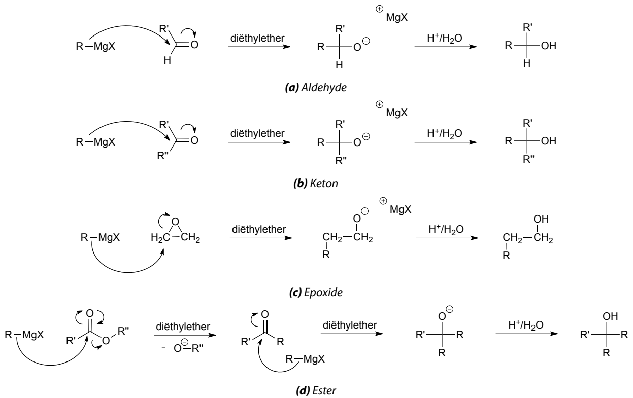
Figuur 5.44 Het mechanisme van de Grignardreacties voor verschillende substraten
