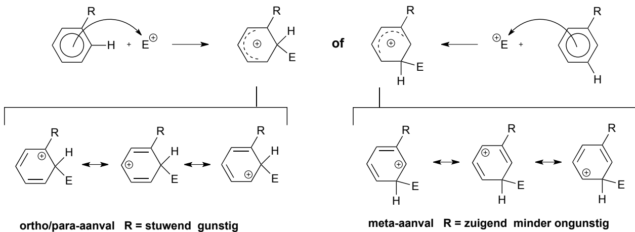
Figuur 5.25 Mechanisme van S_N1Ar
