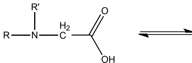
Figuur 4.8 Zwitterionstructuur van EDTA
