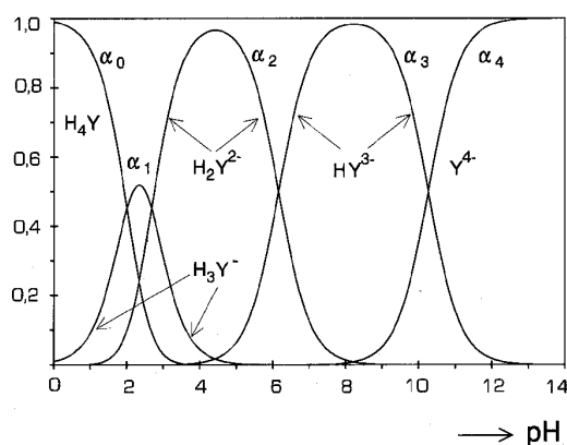
Figuur 4.10 Het distributiediaagram van EDTA
