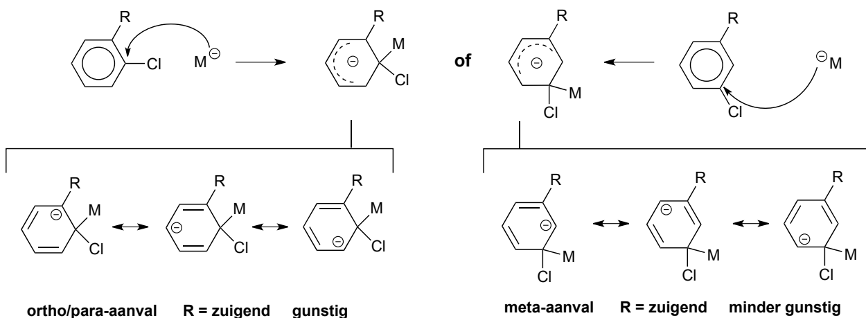
Figuur 5.22 Het richtende effect van substituenten bij aromatische substitutie
