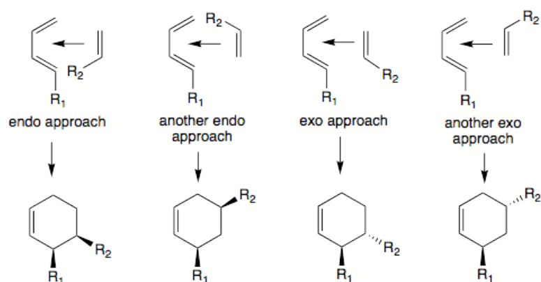
Figuur 5.55 De mogelijke toenaderingen van een diënofiel in termen van endo - en exo -isomeren.
