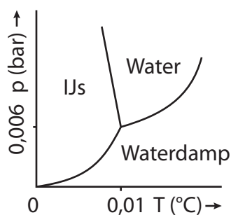
Figuur 4.11 Vereenvoudigd fase-diagram van water
